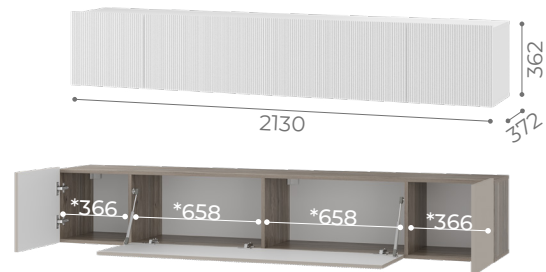
ШКАФ НАВЕСНОЙ ШКН-03
