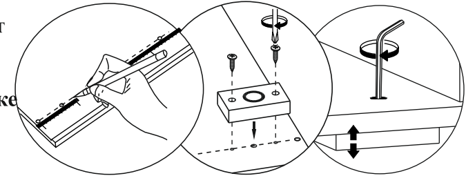
Рис. 3. Установка Опор
