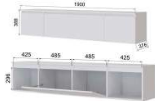
МГТ-2 Тумба ТВ (ВхШхГ) 388х1900х376
