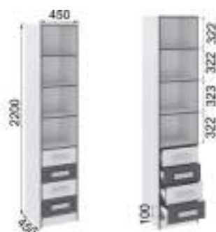
Пенал с ящиками (ВхШхГ) 2200х450х450
