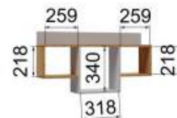
Полка навесная ПНМ-2 (ВхШхГ) 500x900x196
