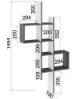
Полка навесная (ВхШхГ) 1464х800х190
