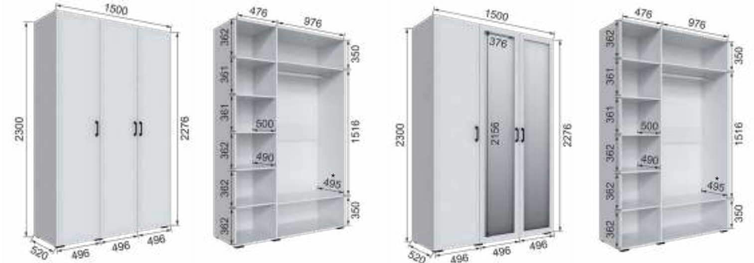
150Ш без зеркала (ВхШхГ) 2300x1500x520
