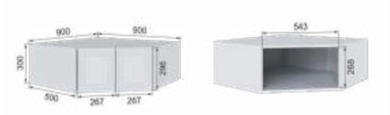
АУС300 (ВхШхГ) 300x900x900
