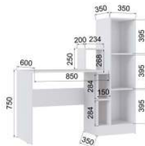
Компьютерный стол СКМ-2 (ВхШхГ) 1350x1350x600
