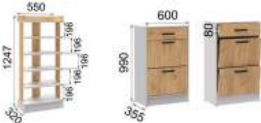
Обувница открытая (ВxШxГ) 1247x550x320
