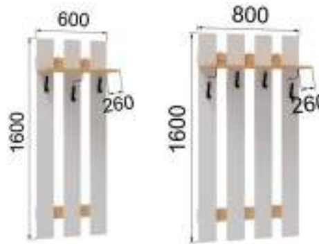
Вешалка 600 (ВxШxГ) 1600x600x292
