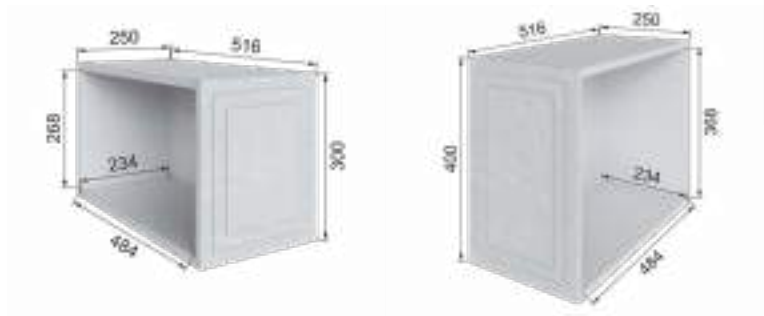
25AT300 (ВхШхГ) 300x250x516
