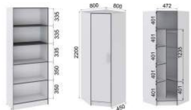
Шкаф угловой (ВхШхГ) 2200х800х800
