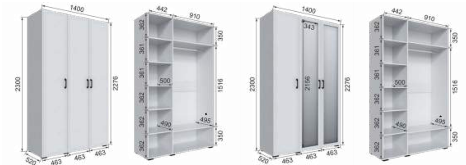
140Ш без зеркала (ВхШхГ) 2300x1400x520
