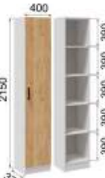
Пенал (ВxШxГ) 2150x400x375
