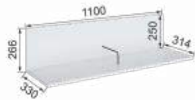
110ГНО-3 (ВхШхГ) 266х1100х330
