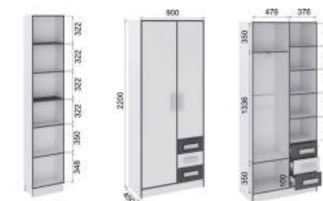
Шкаф торцевой (ВхШхГ) 2200х230х450
