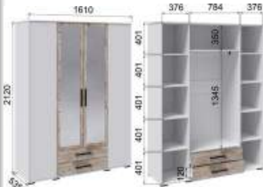
Шкаф 4-х створчатый (ВхШхГ) 2120x1610x535
