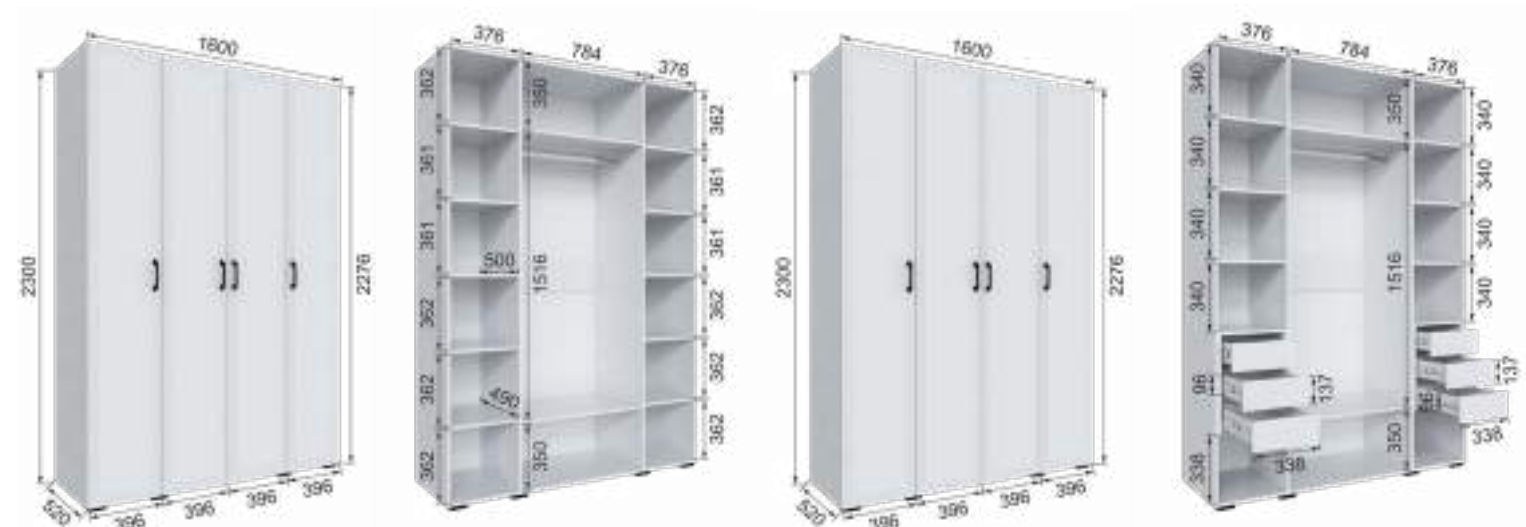
160Ш без зеркала (ВхШхГ) 2300x1600x520
