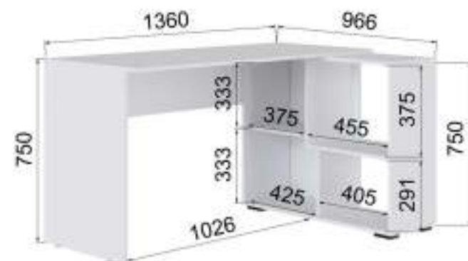
Компьютерный стол угловой СКМУ-4 (ВхШхГ) 750x1360x966
