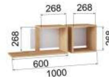
Полка навесная ПНМ-3 (ВхШхГ) 750x600x236/300x1000
