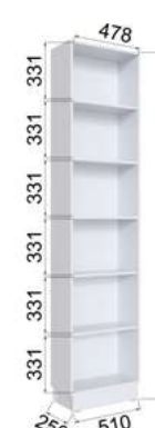
MCSH-22 Шкаф торцевой (ВхШхГ) 2200х510х250
