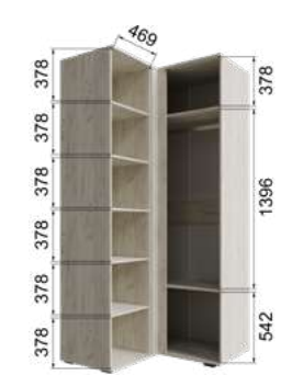
ЛСШ-25 Шкаф угловой (ВхШхГ) 2400х1120х1120
