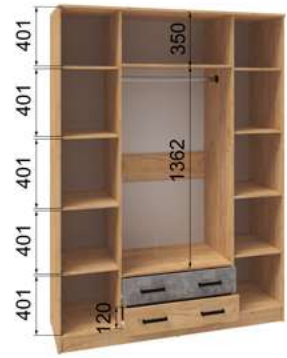
Шкаф 4-х створчатый (ВхШхГ) 2200х1600х540
