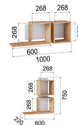
Полка навесная ПНМ-3 (ВхШхГ) 750х600х236/300х1000
