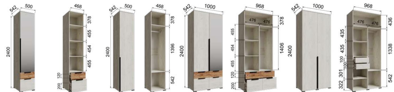
ЛСП-20 Пенал с зеркалом и ящиками (ВхШхГ) 2400х500х542
