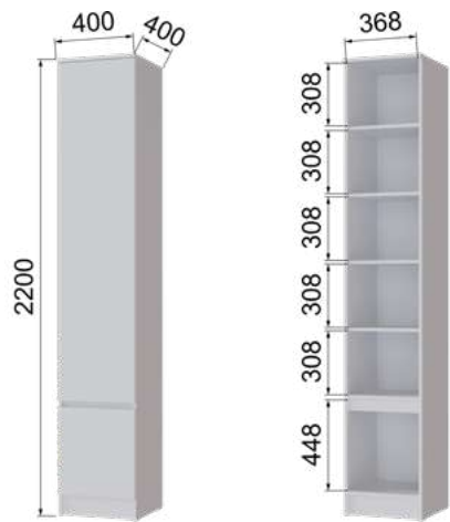
МПП-30 Пенал (ВхШхГ) 2200x400x400
