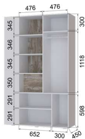
Гардеробная Внутренняя часть левая (ВхШхГ) 2100х1300х450
