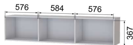
РГТ Тумба ТВ (ВхШхГ) 399x1800x380
