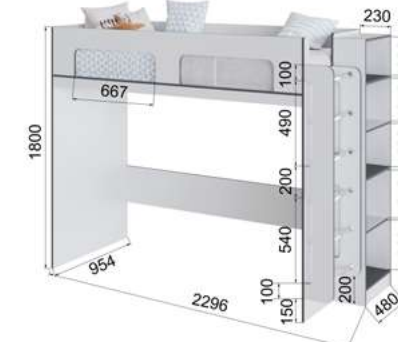
Кровать-чердак (ВхШхГ) 1800х2296х954 Спальные место 2000х900
