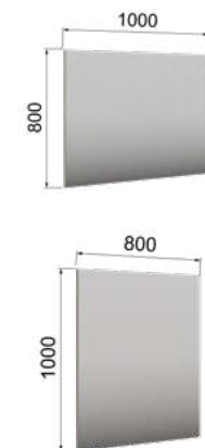
ЛСЗ-20 Зеркало (ВхШхГ) 800/1000х1000/800х20
