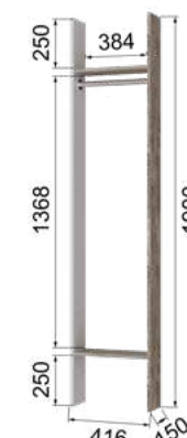
Вешалка (ВхШхГ) 1900х416х150
