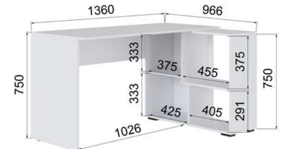
Компьютерный стол угловой СКМУ-4 (ВхШхГ) 750х1360х966
