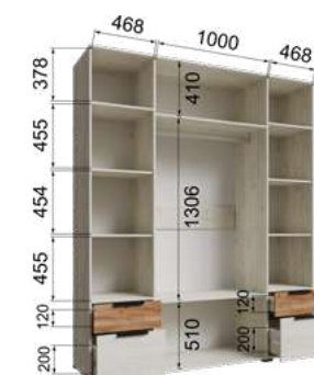
ЛСШ-24 Шкаф 4-х створчатый (ВхШхГ) 2400х2000х542
