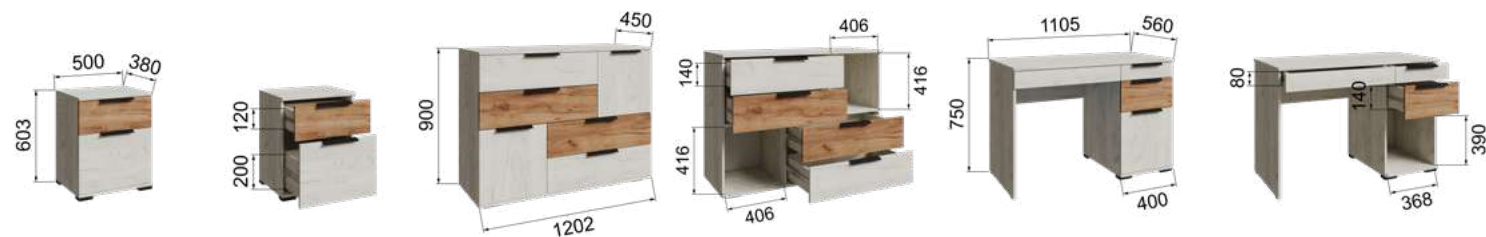
ЛСТ-20 Тумба прикроватная (ВхШхГ) 603х500х380
