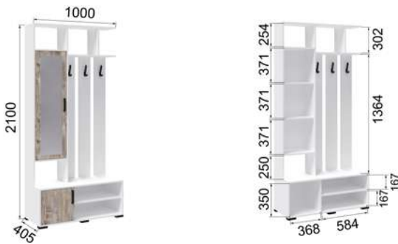
Центральная секция (ВхШхГ) 2100х1000х405
