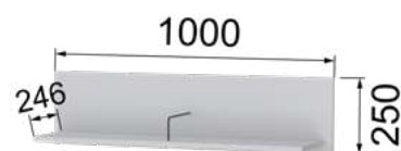
РГН Полка навесная (ВхШхГ) 250x1000x246
