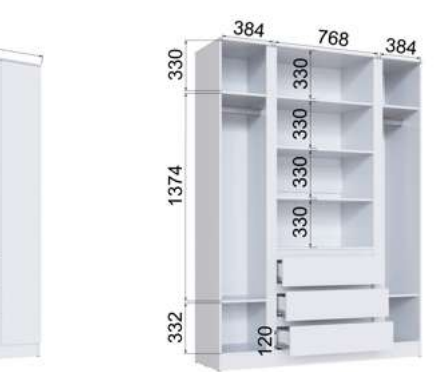
MCSH-25 Шкаф 4-х створчатый (ВхШхГ) 2200х1600х510
