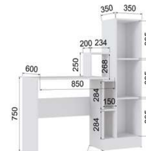
Компьютерный стол СКМ-2 (ВхШхГ) 1350х1350х600
