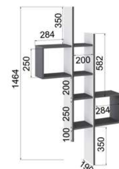
Полка навесная (ВхШхГ) 1464x800x190
