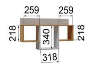
Полка навесная ПНМ-2 (ВхШхГ) 500х900х196
