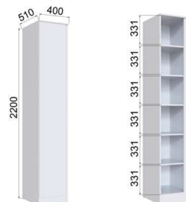
MCP-20 Пенал (ВхШхГ) 2200х400х510
