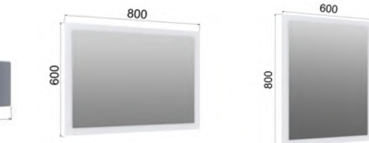
MC3-20 Зеркало (ВхШхГ) 600/800х800/600х20
