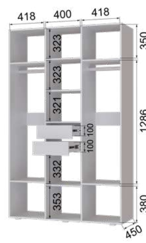
Гардеробная Внутренняя часть правая (ВхШхГ) 2100х1300х450
