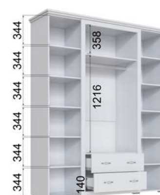
Шкаф 4-х створчатый (ВхШхГ) 2244х1842х550
