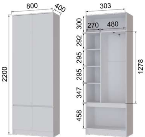
МПСШ-31 Шкаф (ВхШхГ) 2200x800x400
