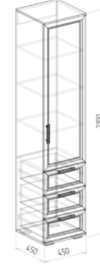
№13* Пенал с ящиками 450
