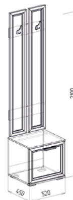
№22* Тумба с вешалкой 450
