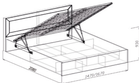
№33/№34 Кровать №1 (подъемная с основанием)
