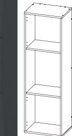
Пенал ЦРК.ОНК.12 431 x 1260 x 304 мм
