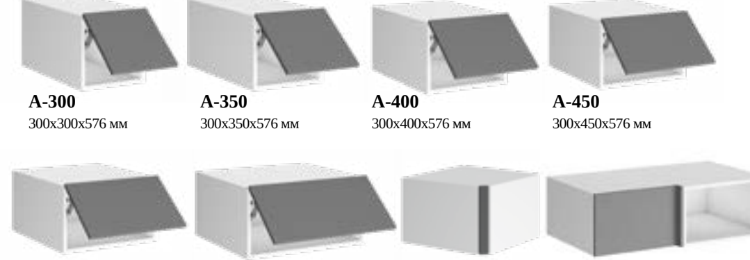
А-300 300x300x576 мм А-350 300x350x576 мм А-400 300x400x576 мм А-450 300x450x576 мм А-500 300x500x576 мм А-600 300x600x576 мм АФ-600У 300x466x466 мм А-1000У 300x997x600 мм
