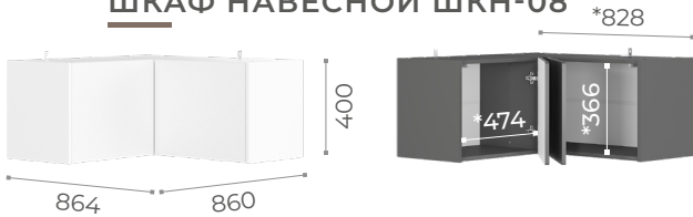
ШКАФ НАВЕСНОЙ ШКН-08
