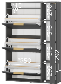
ОБУВНИЦА ТБ-23
