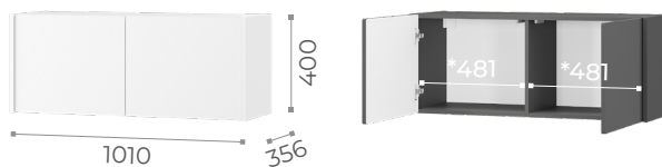
ШКАФ НАВЕСНОЙ ШКН-06
